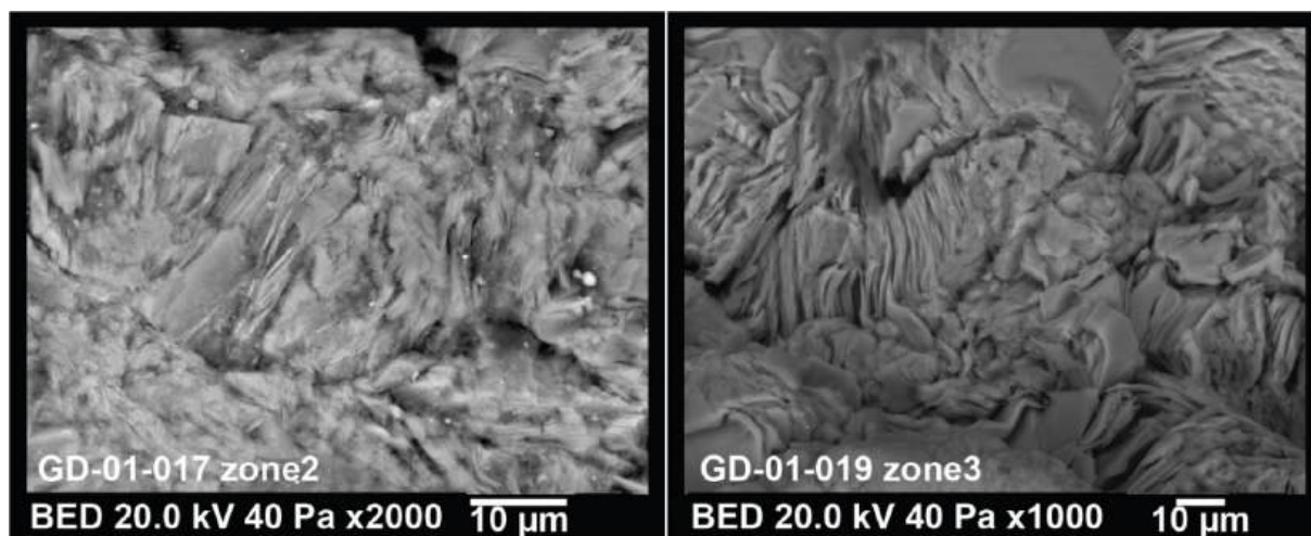
Figure 11. Vues au MEB de la structure en feuillets des artefacts en sudoite, conformément à ce qui est attendu pour un phyllosilicate.
