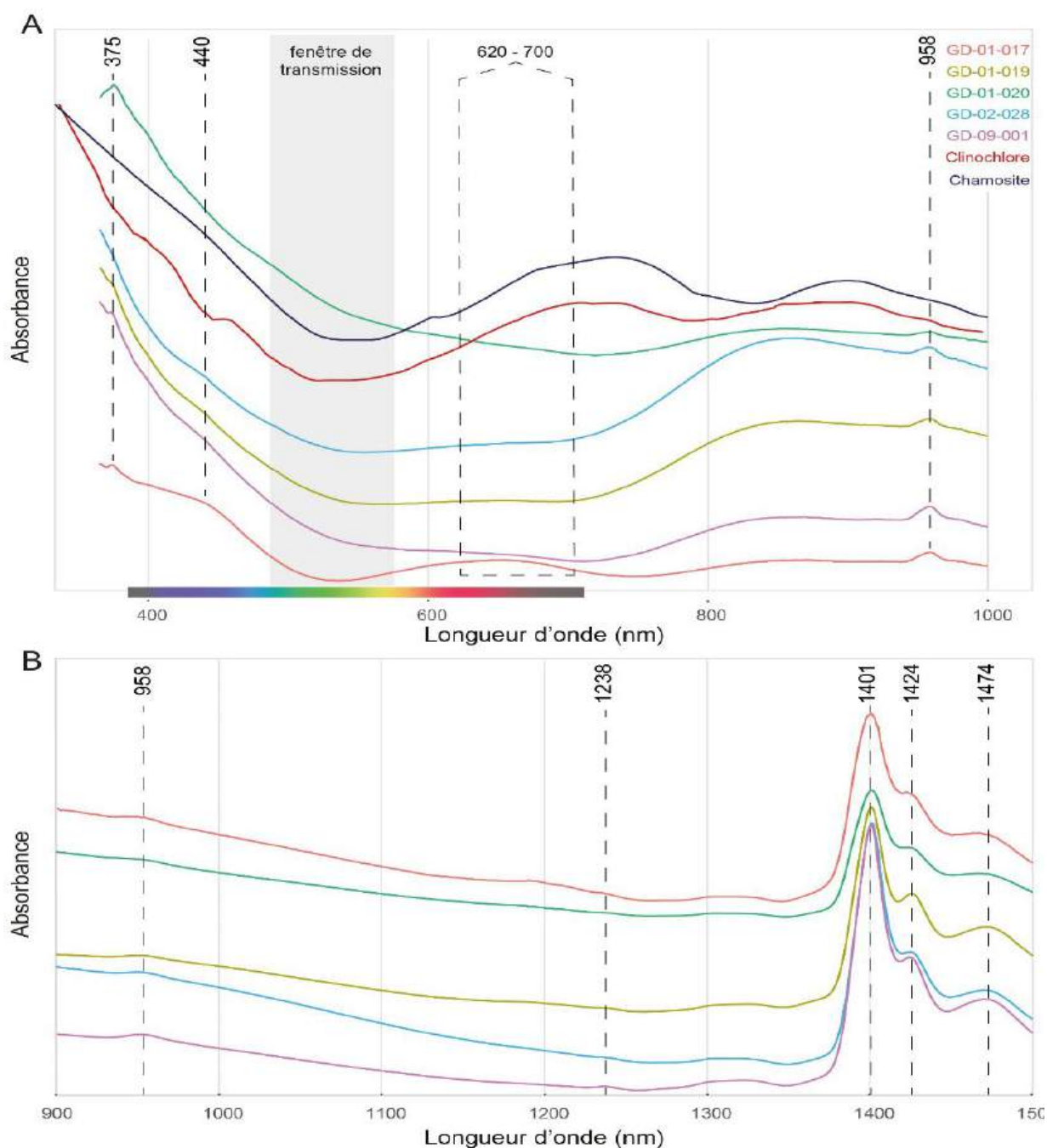
Figure 15. Spectres UV-Vis-NIR obtenus sur les échantillons archéologiques avec le GemmoSphere (A) et le Perkin Elmer avec accessoire 3D et sphère intégratrice(B). Les spectres de clinoclure et de chamosite ont été retracés d'après Bishop et al. (2008 fig. 6) et ne sont pas à l'échelle.
