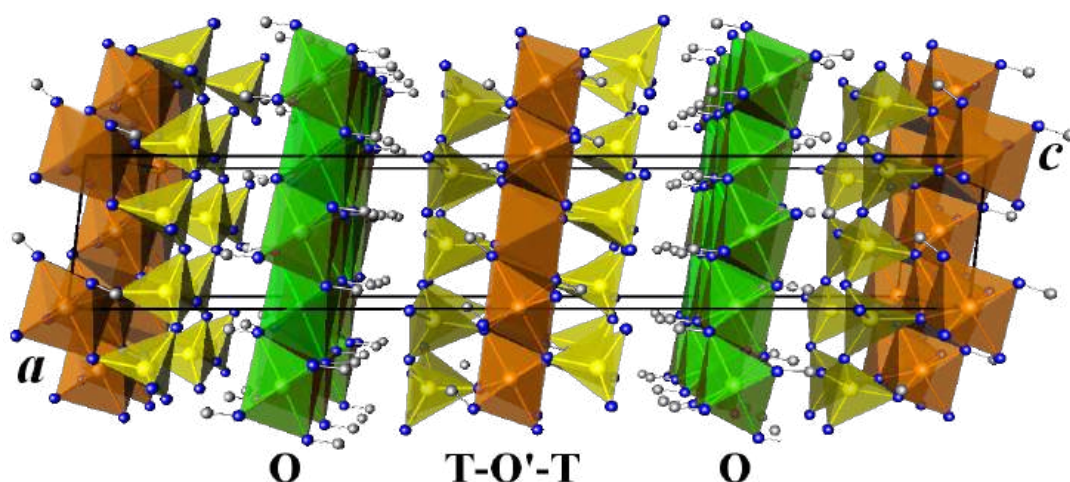
Figure 1. Représentation en perspective de la structure de la sudoite, projetée le long de l'axe b. Jaune : Si, orange : Al, vert : Mg, bleu : O, gris : H. Modifié d'après structure de cookéite (commons.wikimedia CC0),
