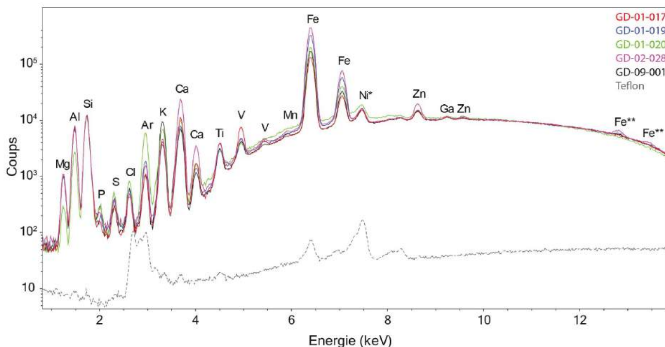
Figure 14. Spectres de fluorescence X en dispersion d'énergie obtenus sur les 5 artefacts exportés, et attribution des différents pics. Le spectre en pointillés correspond au spectre "à vide" de l'appareil de mesure. Les pics notés d'une étoile sont probablement issus de l'appareil en lui-même, tandis que les pics notés de deux étoiles sont des pic d'empilement du fer. L'attention du lecteur est attirée sur le fait qu'il s'agit d'un graphique semi-log permettant d'observer clairement l'ensemble du signal malgré la grande amplitude qui existe entre le nombre de coups des éléments légers et lourds.
