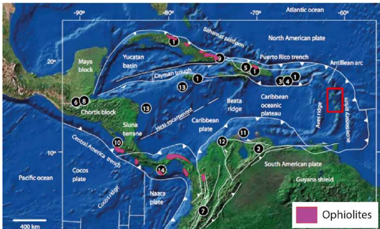
Figure 18. Configuration de la tectonique des plaques et autres faits géologiques majeurs dans la région caribéenne (les numéros se rapportent aux cas d'étude de l'article source) (modifié d'après Garcia-Gasco et al. 2006, 2011). Le cadre rouge indique la localisation des Antilles françaises.
