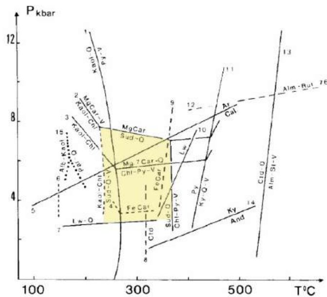
Figure 17. Graphique de stabilités d'une sélection de minéraux métamorphiques d'intérêt pour l'évolution d'une métapélite. La zone de stabilité de la sudoite est colorée en jaune. Chl – chlorite ; Kaol. – kaolinite ; MgCar – Mg-carpholite ; Py – pyrophyllite ; Q – quartz ; Sud – sudoite ; V – H 2 O. Modifié d'après Goffé et al. 1988.
