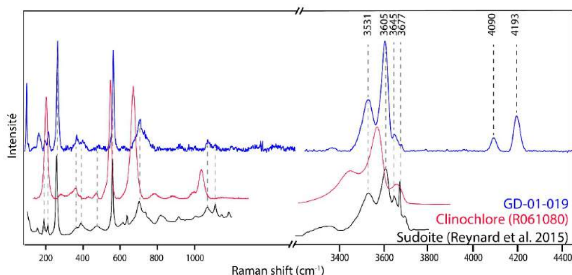
Figure 7. Comparaison entre le spectre Raman obtenu sur l'objet GD-01-019, un spectre Raman de clinoclure issu de la base de données RRUFF, et le spectre redessiné à partir de Reynard et al. 2015 (figure 1). Les spectres sont décalés pour améliorer la lisibilité de la figure.
