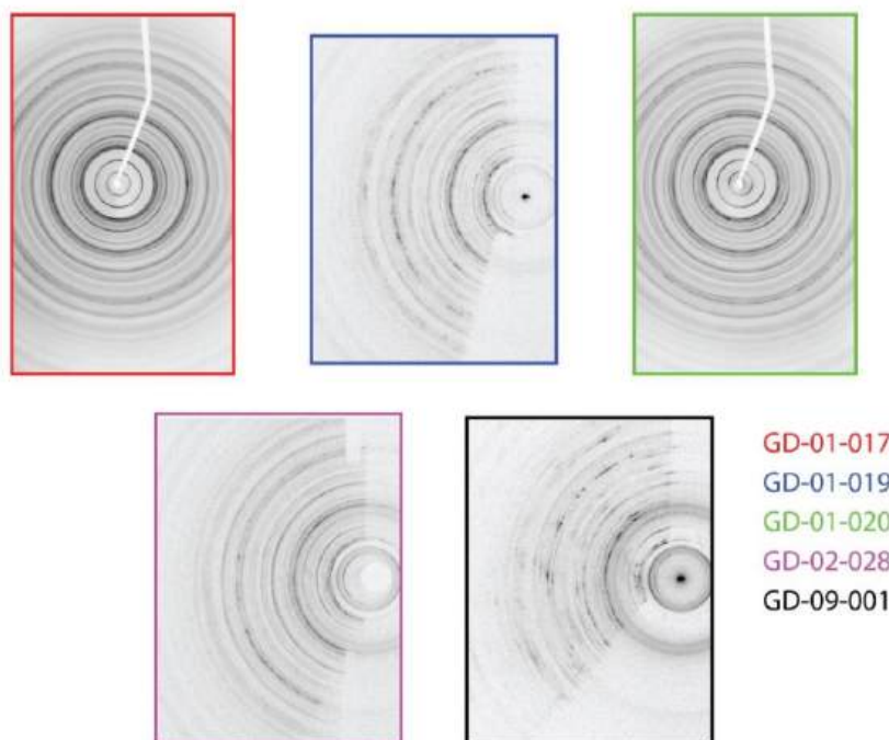
Figure 10. Figures de diffraction obtenues en transmission (GD-01-017 et GD-01-020) et en mode rasant (GD-01-019, GD-02-028 et GD-09-001). L'observation d'anneaux et non de tâches disjointes indique que l'échantillon est polycristallin.
