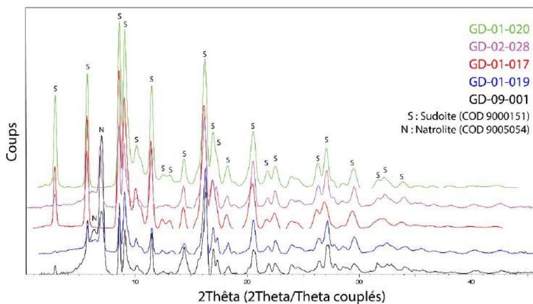
Figure 9. Diffractogrammes obtenus sur les 5 artefacts amérindiens, en transmission ou en faisceau rasant, et attribution des différents pics à la sudoite (S) et la natrolite (N). Les spectres sont décalés pour améliorer la lisibilité de la figure.
