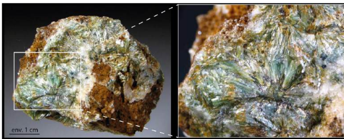
Figure 17. A. Photographie et microphotographie d'un échantillon commercialisé montrant l'existence de nodules fibroradiés plurimillimétriques de sudoite (modifié d'après www.dakotamatrix.com ).
