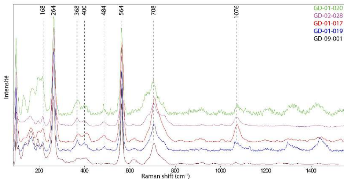
Figure 6. Spectres Raman obtenus au laboratoire sur les artefacts exportés, montrant la répétabilité des mesures. Les spectres sont décalés pour améliorer la lisibilité de la figure.
