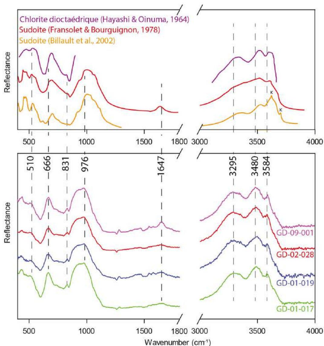
Figure 8. Spectres FTIR issus de la littérature (en haut, retracés à partir des publications) et spectres obtenus avec un équipement ATR sur les objets archéologiques (en bas). K indique d'après l'article original la présence de kaolinite. Les spectres sont décalés pour améliorer la lisibilité de la figure.
