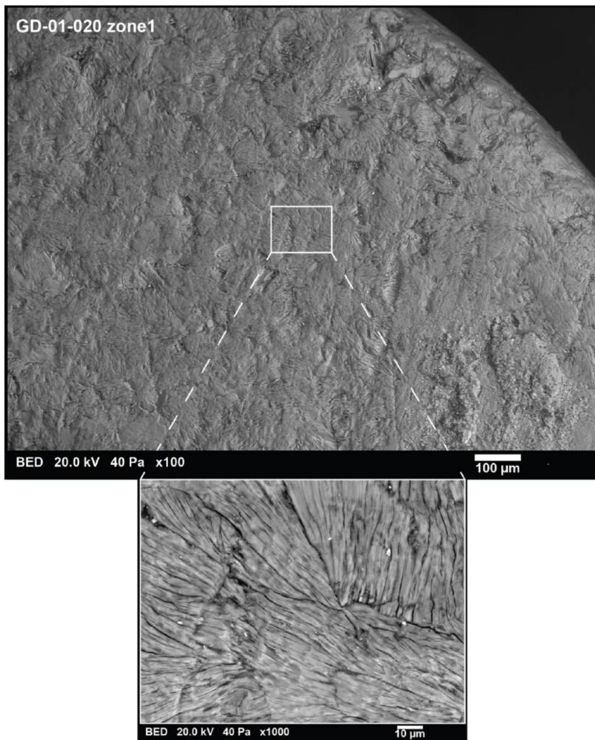
Figure 13. Vues au MEB des différents secteurs multidirectionnels de feuillets et de l'homogénéité du matériau en termes de chimie.
