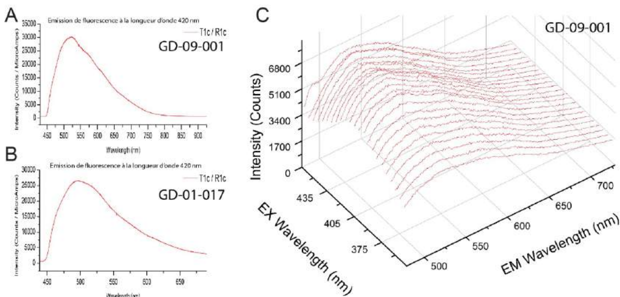
Figure 16. Spectres d'émission de fluorescence à la longueur d'onde 420 nm de l'artefact GD-09-001 (A) et GD-01-017 (B). Spectres d'émission de fluorescence en fonction de la longueur d'onde de l'excitatrice pour GD-09-001 (C).
