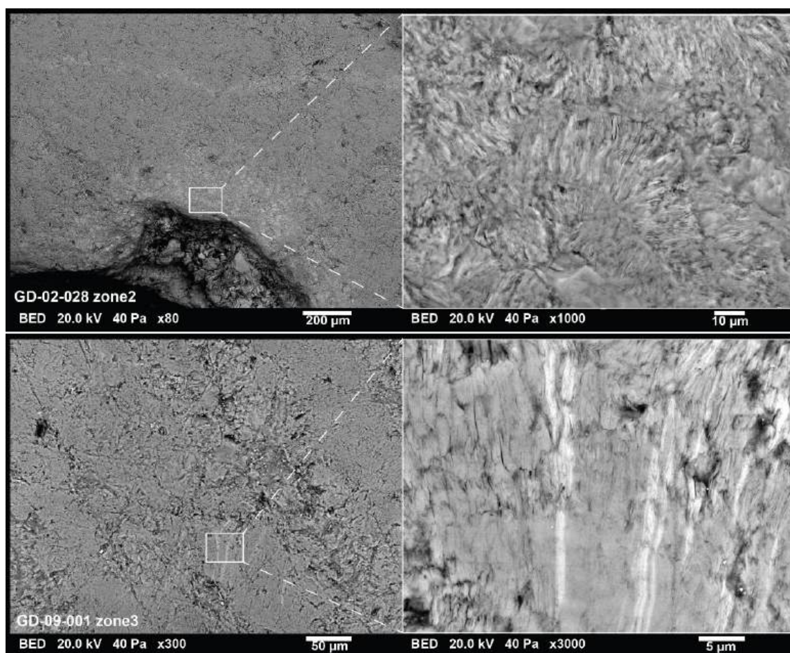
Figure 12. Vues au MEB des feuillets de compositions différentes révélées par des zones plus claires, indiquant une concentration plus importante en éléments lourds.
