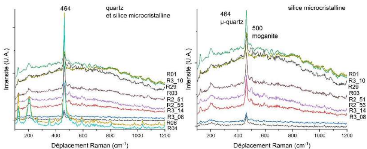
Figure 20. Spectre Raman des silices micro à cryptocristalline, avec ou sans moganite ( 500\text{ cm}^{-1} ) (Exc. 785 nm).
