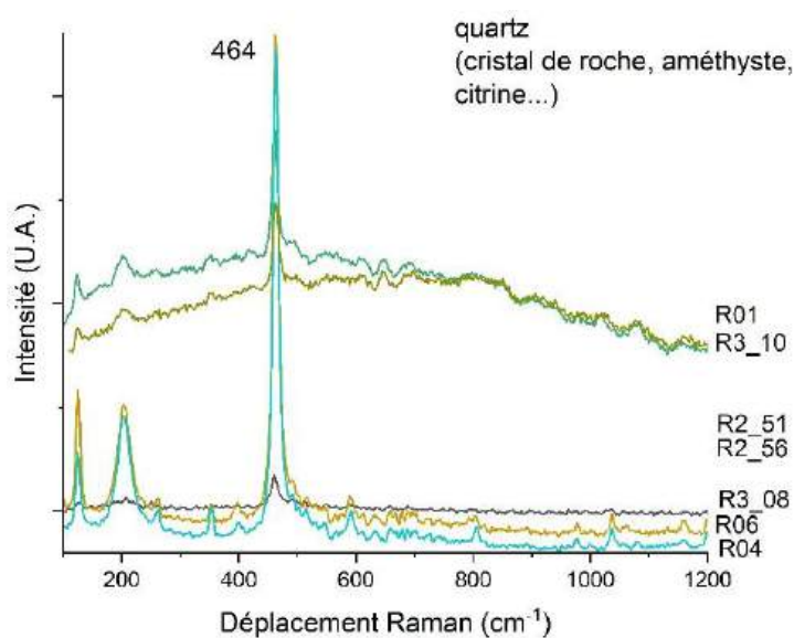
Figure 14. Spectres Raman des quartz monocristallins (cristal de roche et améthyste) (Exc. 785 nm).
