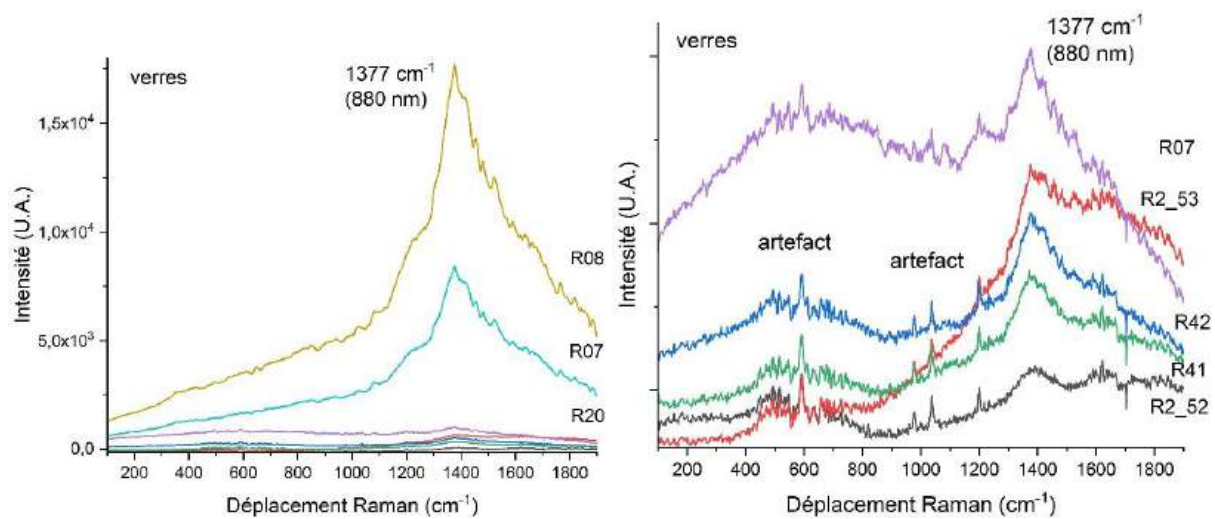
Figure 32. Spectres Raman des verres de la Croix de Castelnau-de-Montmiral (présentant une fluorescence à 880 nm) (Exc. 785 nm).
