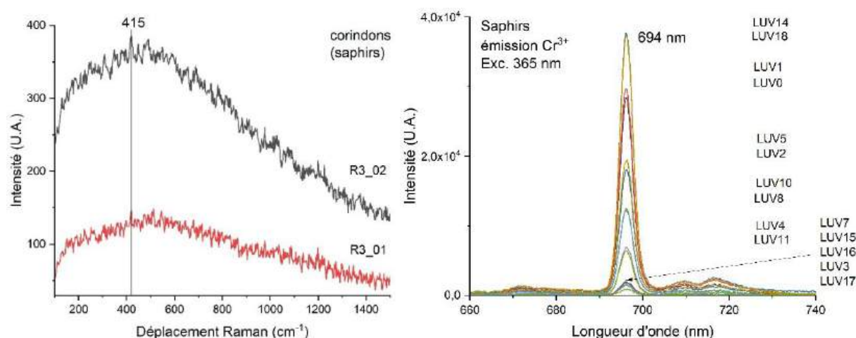
Figure 26. a) Spectres Raman de corindons bleus (saphirs) ; b) Spectres de photoluminescence du chrome \text{Cr}^{3+} des corindons bleus (saphirs) responsable de l'émission rouge à 694\text{ nm} (Exc. UV 365\text{ nm} ).
