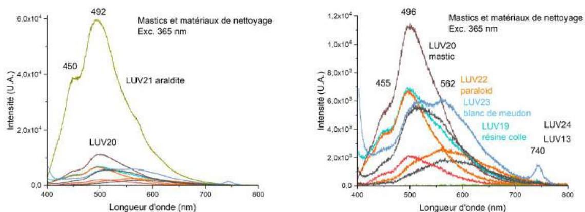
Figure 43. Spectres de photoluminescence des mastics de fixation et de la résine colle, comparés à des références (Araldite, Paraloïd et blanc de Meudon) (exc. UV 365 nm).
